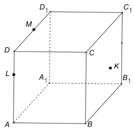
K \in BB_1C_1
