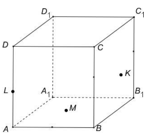
K \in BB_1C_1 M \in ABC
