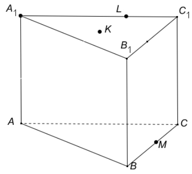
K \in A_1B_1C_1
