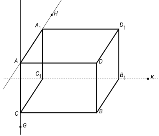
K \in BB_1C_1 M \in ABC
